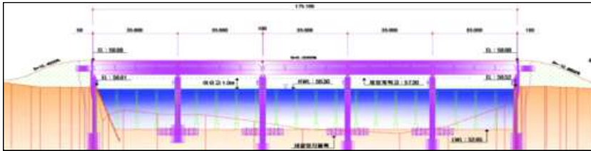
&lt;당초 설계안: 교량(접속도로 종단경사 11%) &gt;
