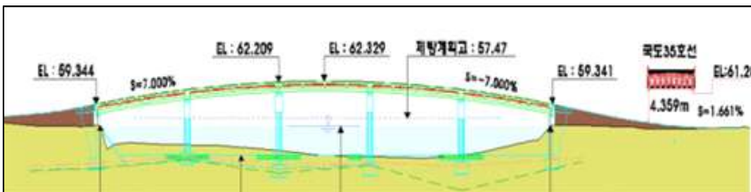
&lt;설계보완 후: 계획홍수위 조정 및 교량 접속도로 종단경사 조정(7%) &gt;
